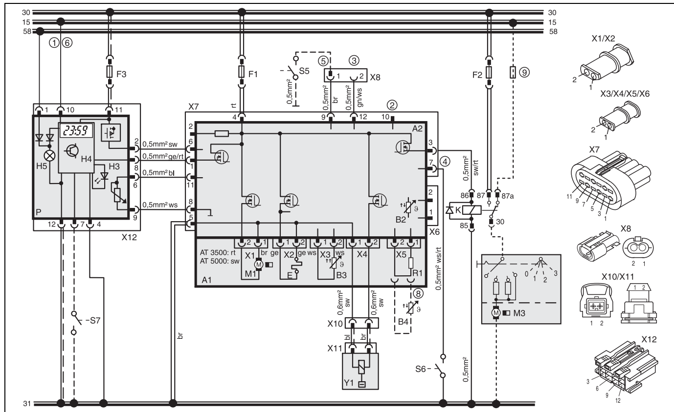
Fig. 32: Esquema eléctrico del sistema Air Top 3500 ST y Air Top 5000 ST, 12V/24V con reloj combinado y soplador del vehículo; para la leyenda, véanse las páginas 64 y 65
