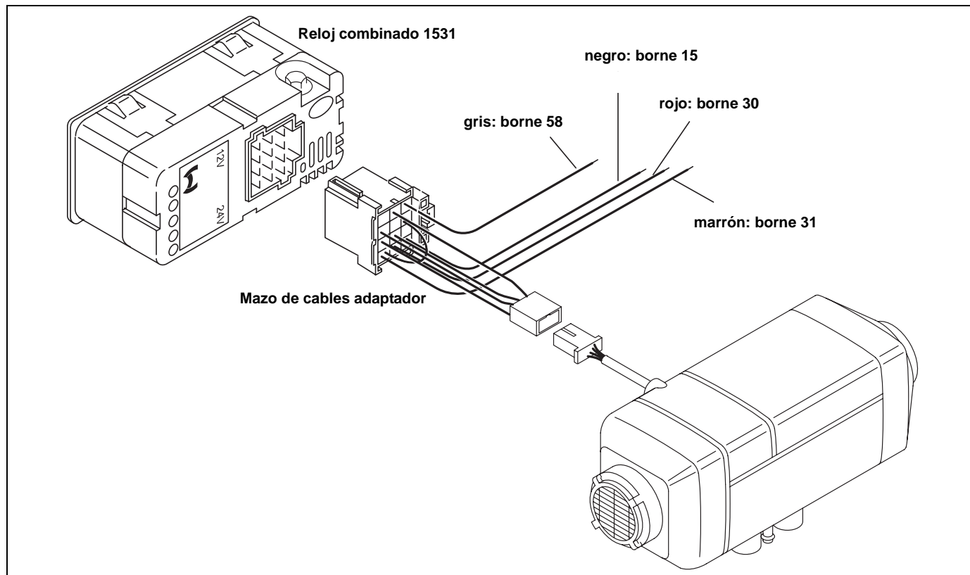
Fig. 30: Esquema de conexiones Air Top 3500 ST y Air Top 5000 ST con reloj combinado
