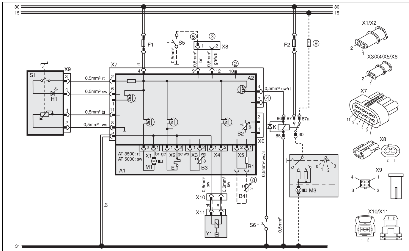
Fig. 31: Esquema eléctrico del sistema Air Top 3500 ST y Air Top 5000 ST, 12V/24V con elemento de mando y soplador del vehículo; para la leyenda, véanse las páginas 64 y 65
